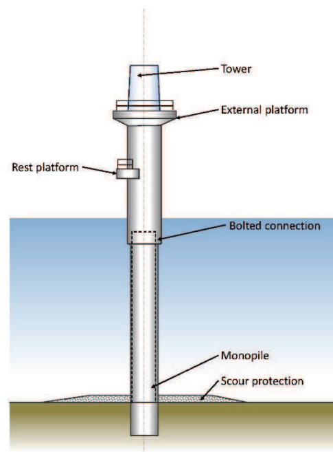
Monopile
