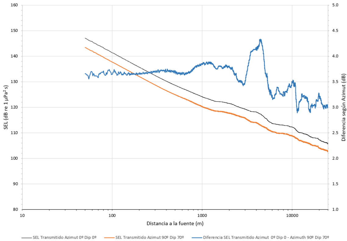
Figura 26. SEL recibido (RL). CAN_100-108. Azimut 0° vs 90° Filtro HF (alta frecuencia)
