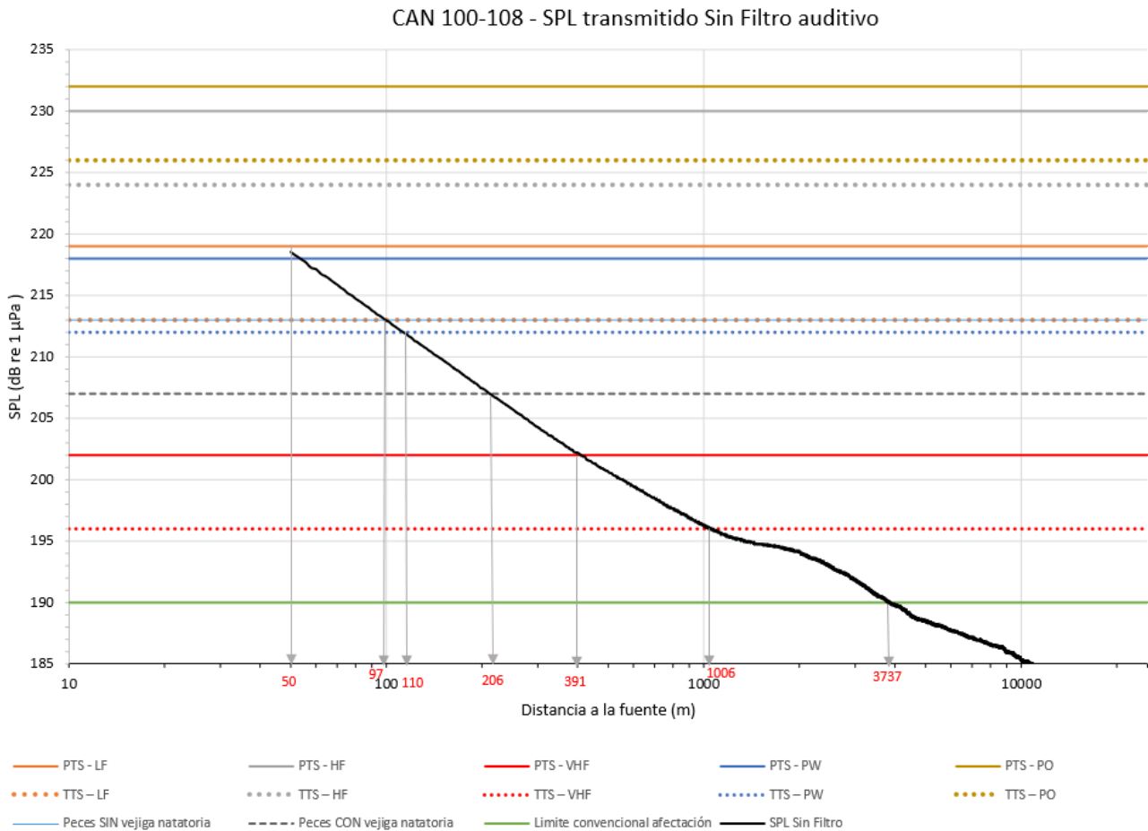
Figura 50. Ejemplo de comparación entre los valores de SPL peak TOTAL y los diferentes umbrales para determinar las distancias correspondientes (CAN_100-108. Azimut 90° - Dip 70°, Suelos AB-GB)
