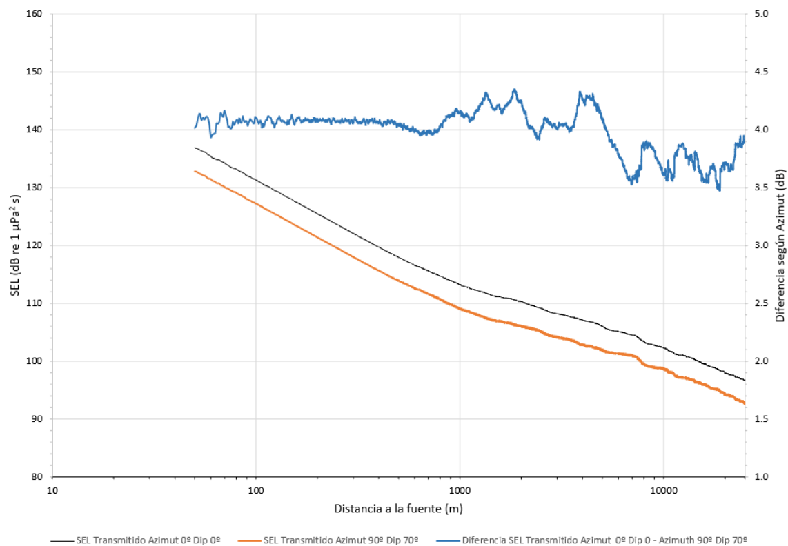
Figura 39. SEL recibido (RL). CAN_114. Azimut 0° vs 90° Filtro VHF (muy alta frecuencia)
