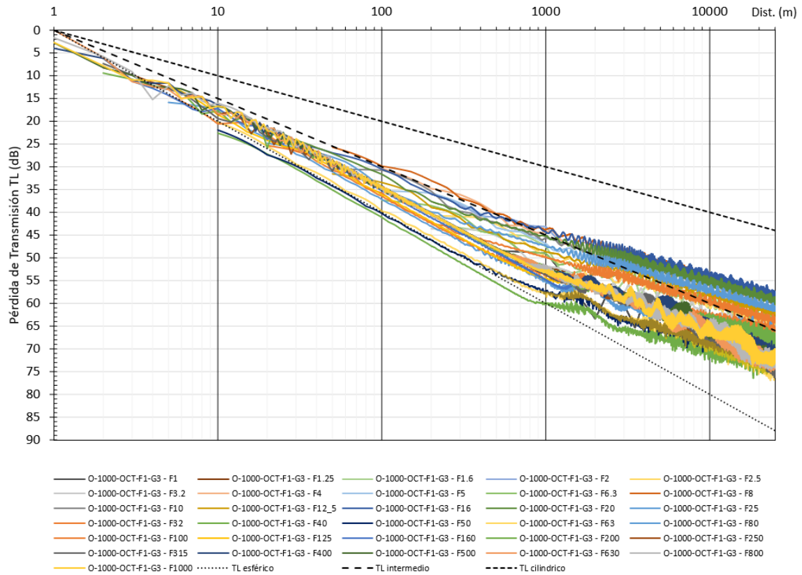
Figura 14. Pérdida de Transmisión mínima en la vertical TL_V para el área CAN_114, con la condición más conservativa del análisis de sensibilidad (Fangos F1 y Gravas subyacentes G3)
