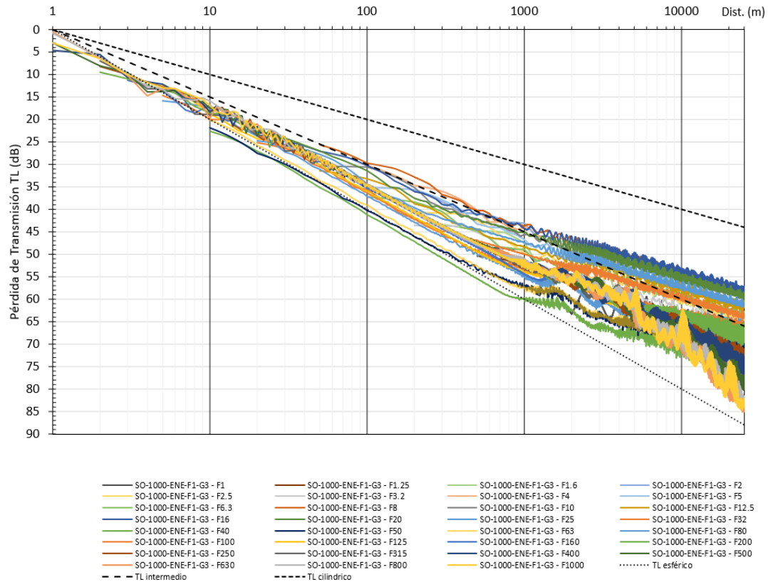
Figura 12. Pérdida de Transmisión mínima en la vertical TL_v para el área CAN_100-108, con la condición más conservativa del análisis de sensibilidad (Fangos F1 y Gravas subyacentes G3)
