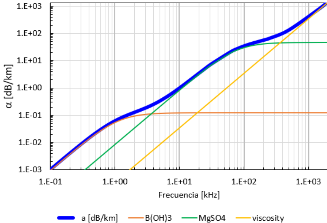
Figura 2. Pérdidas por absorción en función de la frecuencia según la dominancia del Ácido Bórico (B(OH) 3 ), moléculas de Sulfato de Magnesio (MgSO 4 ) y Viscosidad.
