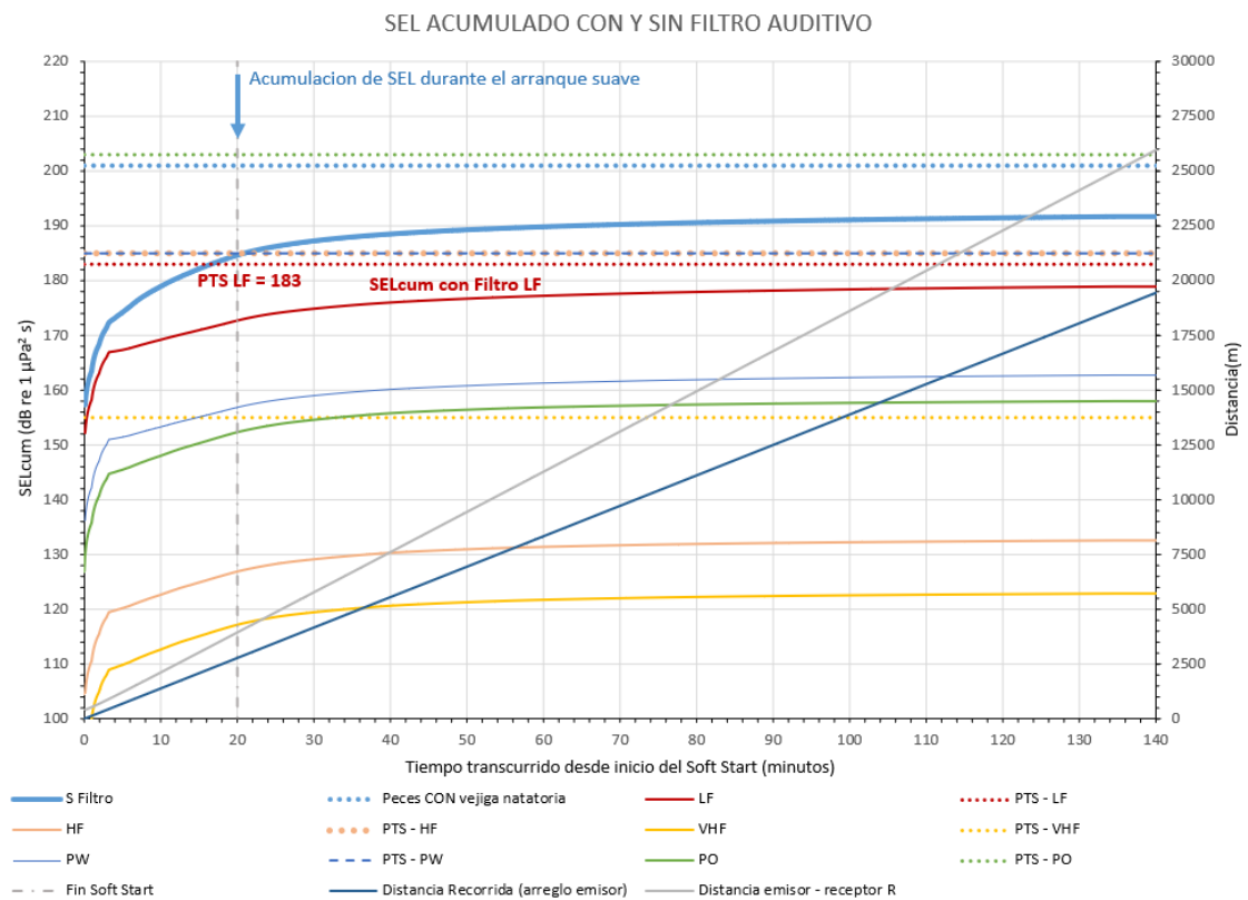
Figura 63. CAN_114. SEL acumulado. Soft Start 20 minutos. Posición inicial del receptor a 400 m del emisor, perpendicular a la línea de avance en el punto de arranque del Soft Start. Azimut movimiento del receptor 90° a 2 m/s.
