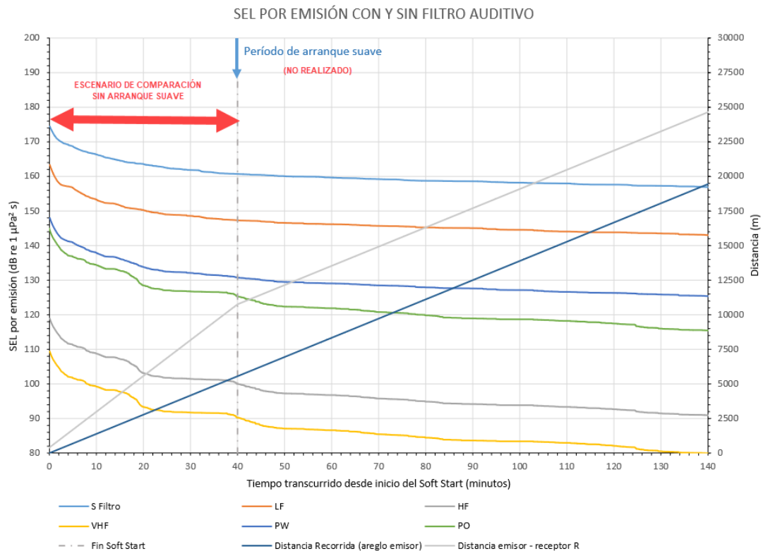
Figura 54. CAN_100-108. SEL recibido por cada emisión. Simulación de comparación SIN Soft Start. Azimut movimiento del receptor 180° a 2 m/s durante 40 minutos.
