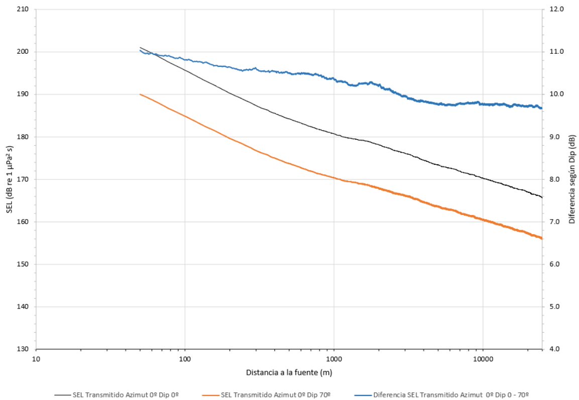
Figura 49. SEL recibido (RL). CAN_100-108. Azimut 0° Dip 0°-70° Sin Filtro. Verificación suelo AB-GB
