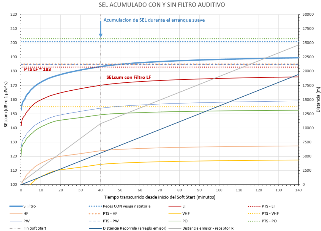
Figura 53. CAN_100-108. SEL acumulado. Soft Start 40 minutos. Azimut movimiento del receptor 180° a 2 m/s durante el Soft Start únicamente.
