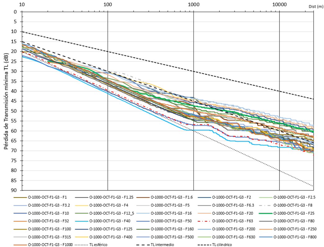
Figura 14. Pérdida de Transmisión mínima en la vertical TL_V para el área CAN_114, con la condición más conservativa del análisis de sensibilidad (Fangos F1 y Gravas subyacentes G3)
