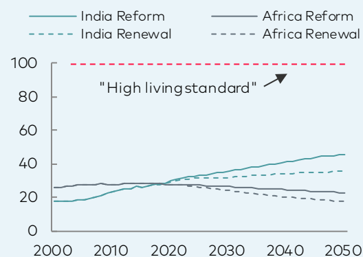
Energy demand per capita
